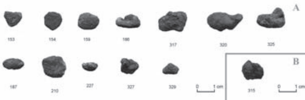
Fig. 2 – Castro da S. Guia de Baiões, evidências de produção de bronze: A - Nódulos de redução em bronze; B - Escoria com vestígios de malaquite e cassiterite (sg. Figueiredo, et al. 2010a: fig. 3 adaptada).
